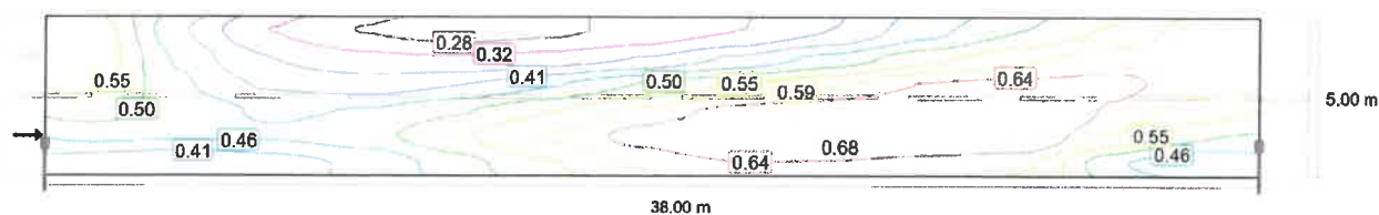
Observator 1: Valoarea de întreţinere, densitatea luminii cu carosabil uscat [cd/m 2 ] (Linii Isolux)
